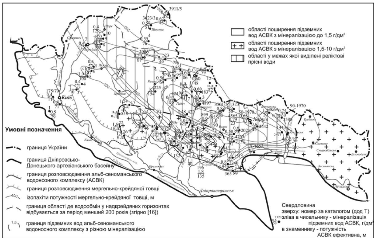
Рис 2. Схематична карта поширення мергельно-крейдяної товщі і реліктових прісних вод у альб-сеноманському водоносному комплексі Дніпровсько-Донецького артезіанського басейну. Масштаб 1:5 300 000. / за даними В. М. Шестопалова, Н. І. Дробнохода, В. І. Лялько та ін./
