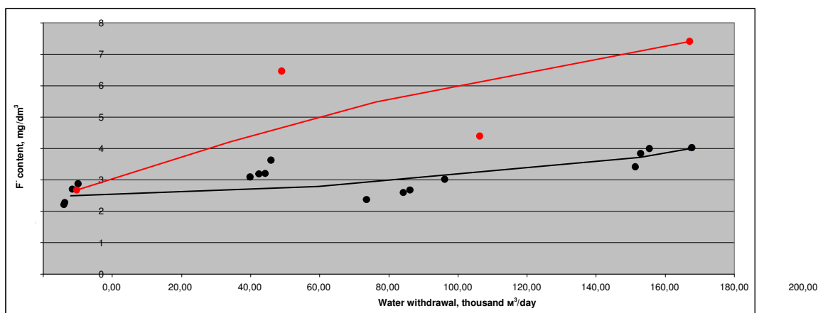
Рис. 2. Кореляційний зв'язок між вмістом F у підземних водах та показником водовідбору на водозаборах № 1 (точки та лінія тренду червоного кольору) та №№ 2-5 (точки та лінія тренду чорного кольору) м. Полтава
