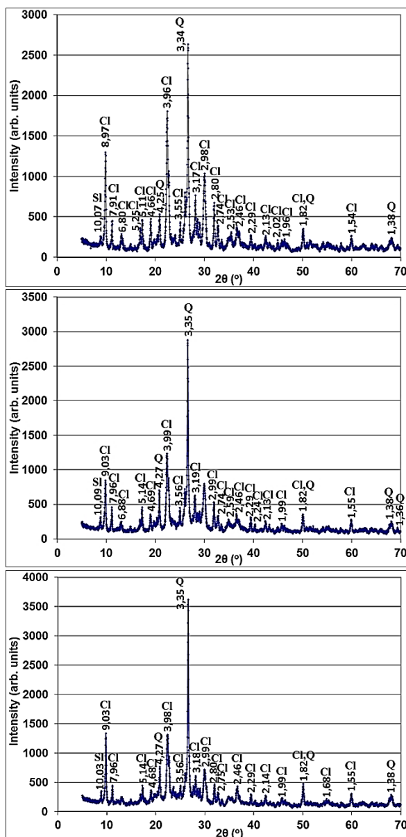
Рис. 1 Дифрактограми цеолітів Сокирницького родовища: А – природного; Б – модифікованого NaOH; В – модифікованого HCl. Q – кварц, Sl – слюда; Cl – клиноптилоліт.
