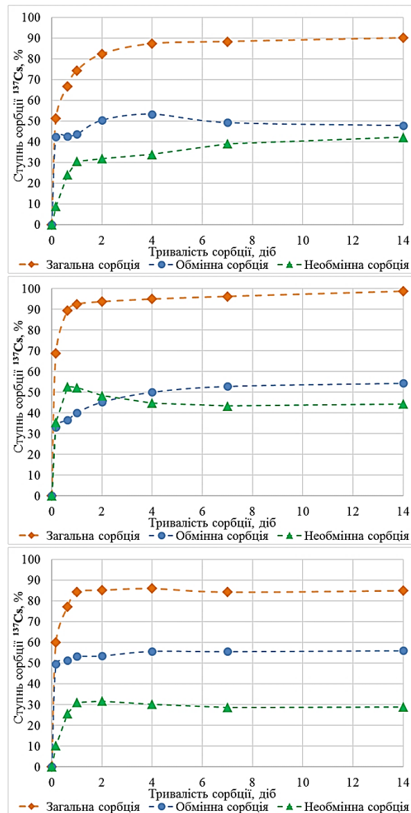
Рис. 2 Сорбція ^{137}\text{Cs} цеолітами Сокирницького родовища: А – природного; Б – лужномодифікованого; В – кислотномодифікованого.
